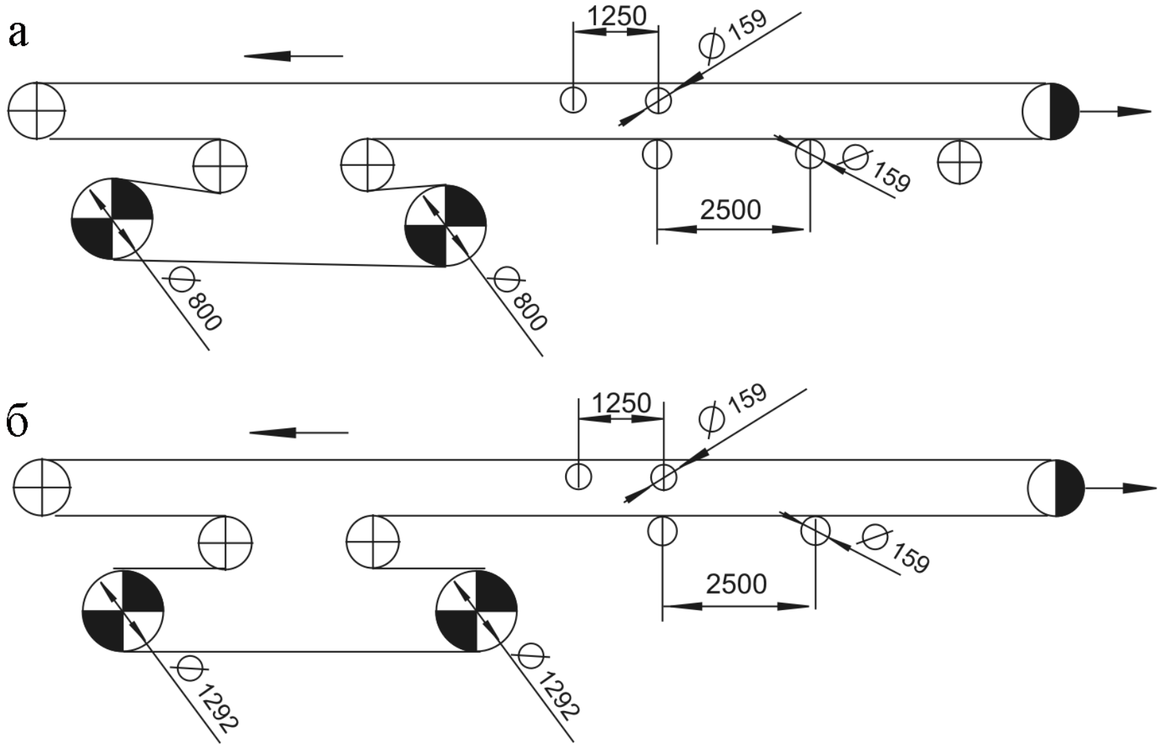
Схеми конвеєрів Олександрійського машинобудівного заводу зі стрічкою шириною 1200мм: а – 1ЛУ120; б – 2ЛУ120А; 2ЛУ120Б
