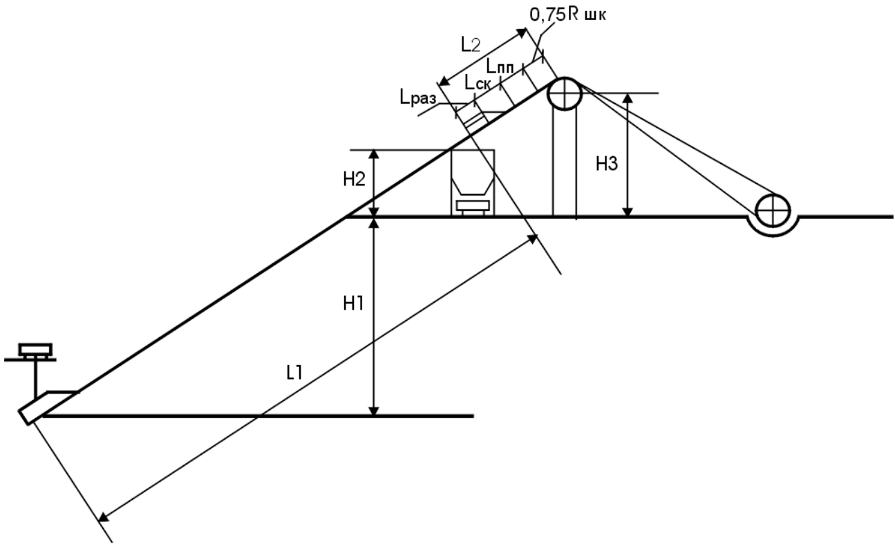
Рис 4.1 Схема двосудиної похилої підйомної установки кар'єру
